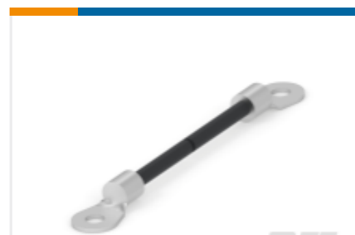
TE Part #1337669-1 7.54MM CSA BRAID M5 - M5 100MM
