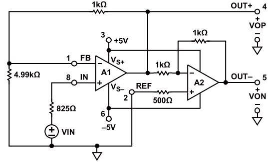
图48. 双电源、 G = 2.4 、单端转差分放大器
