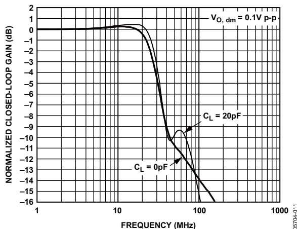
图12. 不同容性负载下的小信号频率响应
