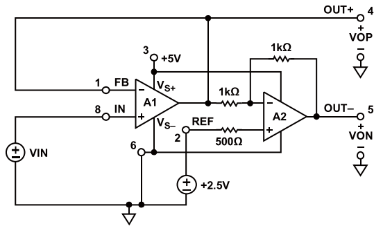
图49. +5V单电源、 G=2 单端转差分放大器
