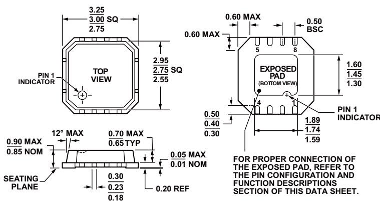
图59. 8引脚引脚架构芯片级封装[LFCSP_VD] 3 mm x 3 mm, 超薄体, 双列引脚(CP-8-2) 图示尺寸单位: mm
