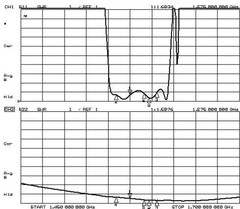
VSWR
