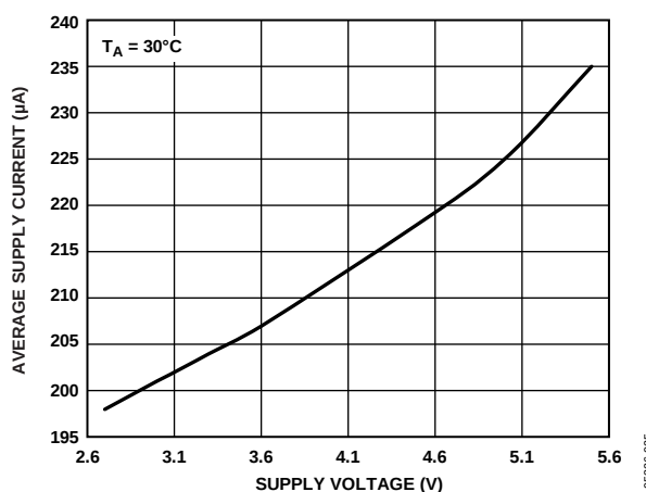
图7. 30°C时平均工作电源电流与电源电压的关系
