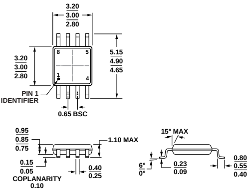
图23. 8引脚超小型封装[MSOP] (RM-8) 图示尺寸单位: mm
