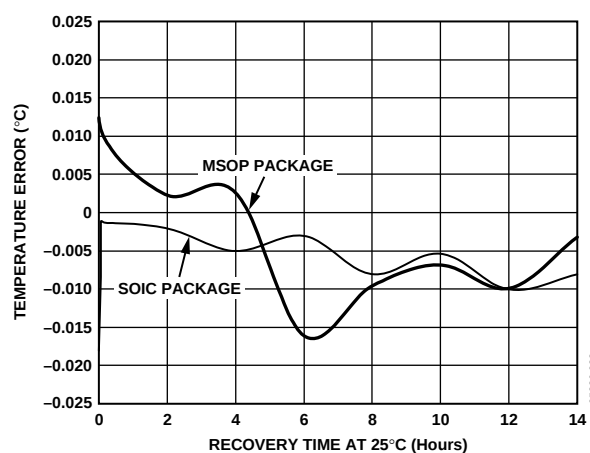
图10. 热冲击响应
