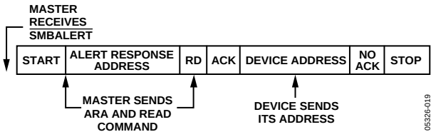
图20. ADT75响应SMBALERT ARA
