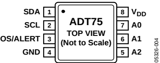
图4. 引脚配置
