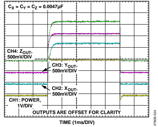
图22. 典型开启时间( V_s = 3V )
