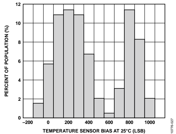
图27. 25°C时的温度传感器响应, V_S = 2 V
