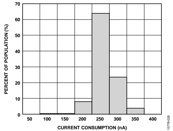
图26. 25°C时的功耗, 唤醒模式, V_S = 2 V
