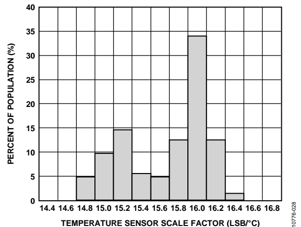
图28. 温度传感器比例因子, V_S = 2 V
