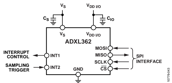
图45. 利用INT2引脚触发同步采样
