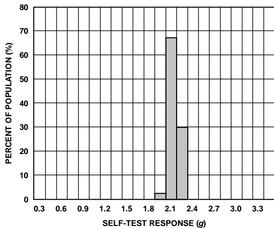
图17. Z自测数据值( V_S = V_{DDIO} = 3.3\text{ V} , 25^\circ\text{C} )
