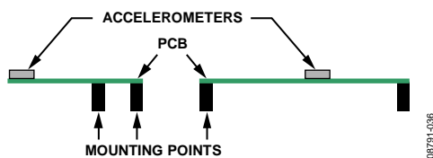
图31. 错误放置的加速度计
