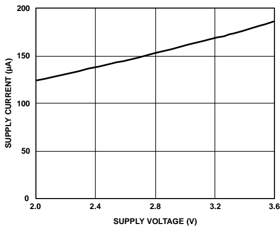
图20. 25^\circ\text{C} 时的电源电流与电源电压的关系
