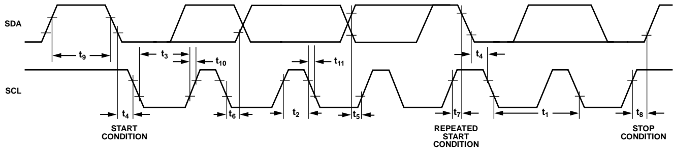
图28. I 2 C时序图
