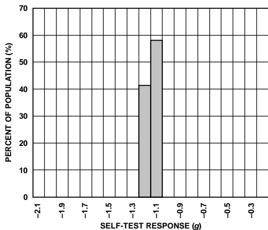
图16. Y自测数据值( V_S = V_{DDIO} = 3.3\text{ V} , 25^\circ\text{C} )
