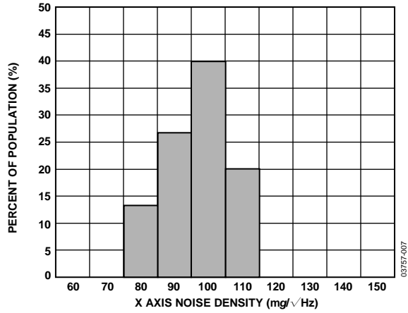
图12. 25°C时的X轴噪声密度
