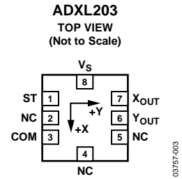
图4. ADXL203引脚配置
