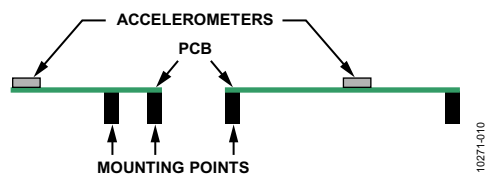
图59. 错误放置的加速度计
