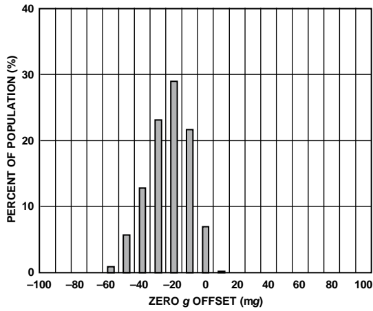
图4. 25°C时的X轴0 g偏移, V_s = 2.5 V
