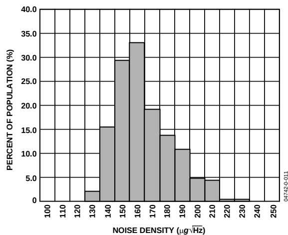
图13. 25°C时的Y轴噪声密度
