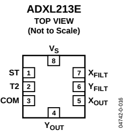
图22. ADXL213 8引脚CLCC
