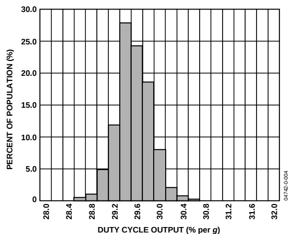
图5. 25°C时的X轴灵敏度
