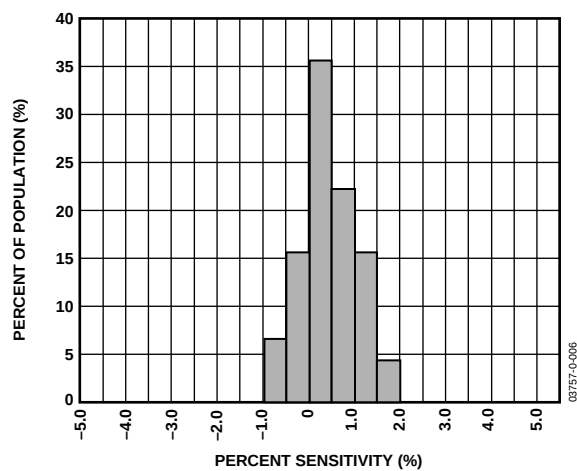
图14. Z与Y的跨轴灵敏度
