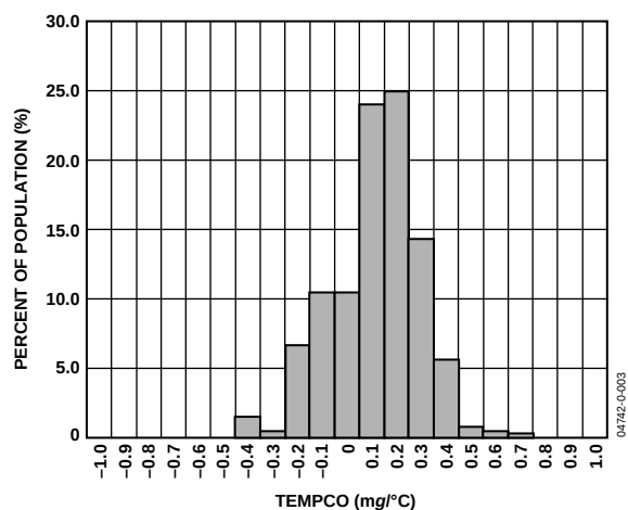
图4. X轴0 g偏置温度系数
