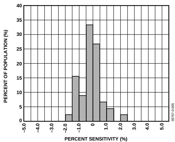
图11. Z与X的跨轴灵敏度
