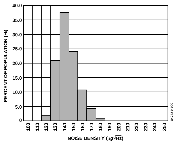
图10. 25°C时的X轴噪声密度
