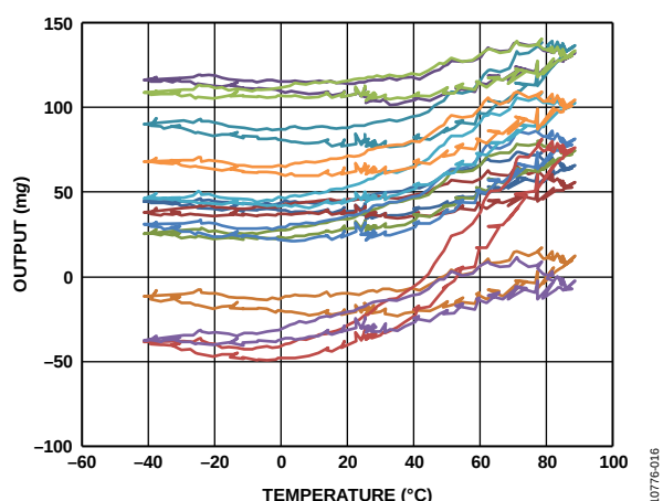
图16. Z轴0 g偏移与温度的关系—16个器件焊接到PCB, ODR = 100 Hz, V_s = 2\text{ V}
