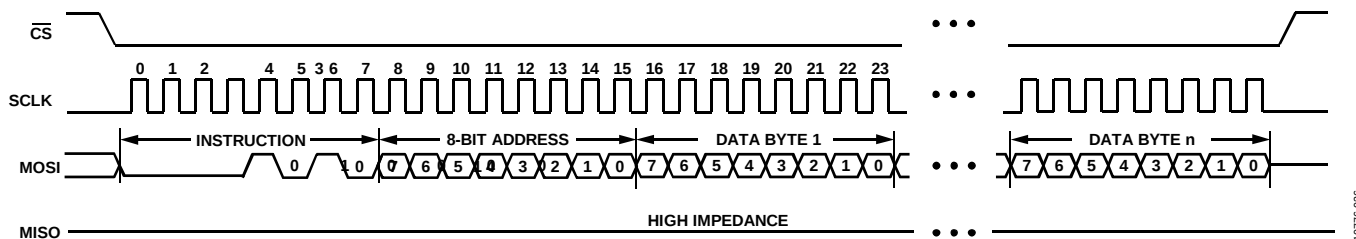
图39. 突发写入
