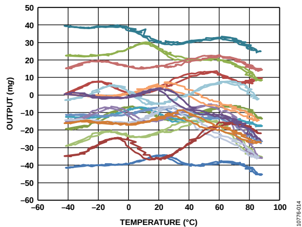
图14. X轴0 g偏移与温度的关系—16个器件焊接到PCB, ODR = 100 Hz, V_s = 2\text{ V}
