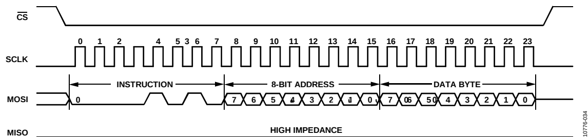
图37. 寄存器写入
