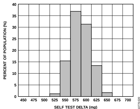
图20. 25°C时的X轴自检响应, V_s = 2 V
