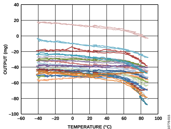
图15. Y轴0 g偏移与温度的关系—16个器件焊接到PCB, ODR = 100 Hz, V_s = 2\text{ V}
