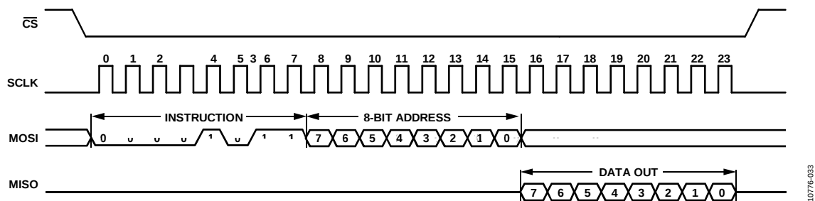
图36. 寄存器读取
