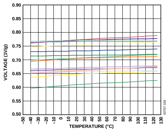
图16. 自测响应与温度的关系
