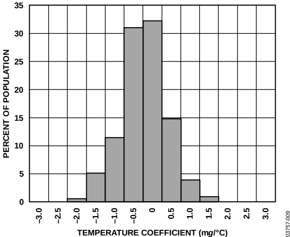
图29. Y轴0 g偏置温度系数
