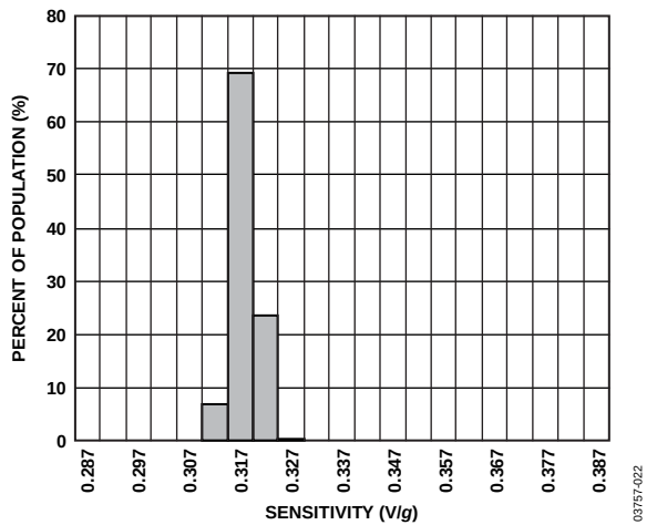
图24. 25°C时的Y轴灵敏度
