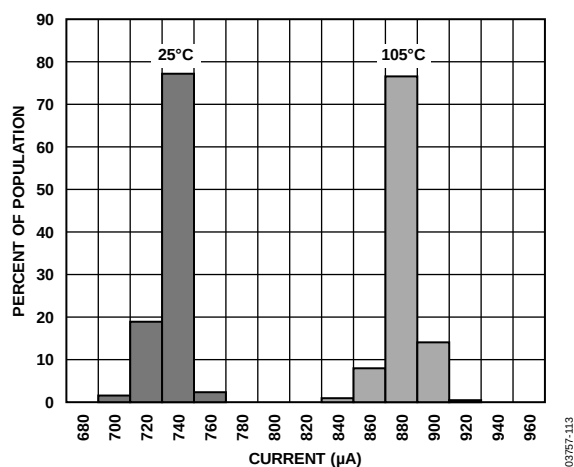
图34. 电源电流与温度的关系
