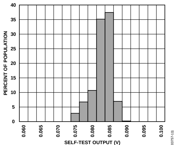
图31. 25°C时的X轴自测响应
