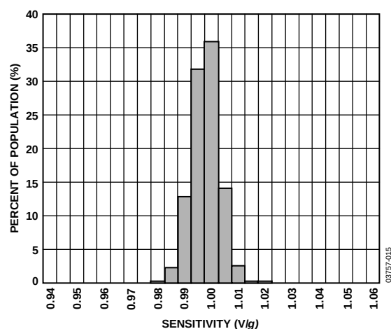
图10. 25°C时的Y轴灵敏度
