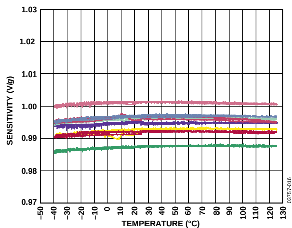
图13. 灵敏度与温度的关系；器件焊接到PCB
