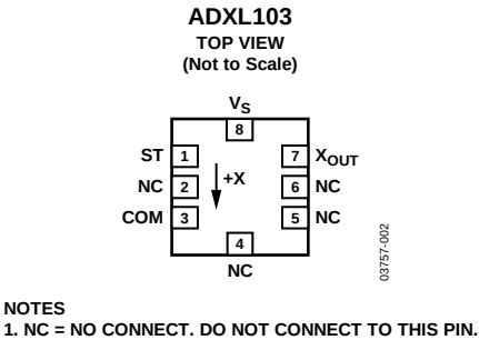
图3. ADXL103引脚配置
