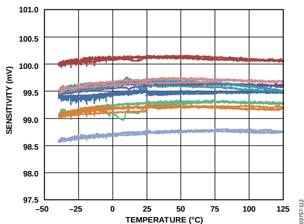
图32. 灵敏度与温度的关系；器件焊接到PCB
