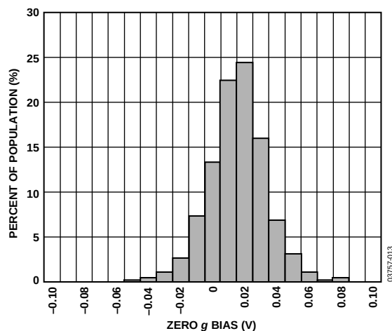
图8. 25°C时相对理想值的Y轴0 g偏置
