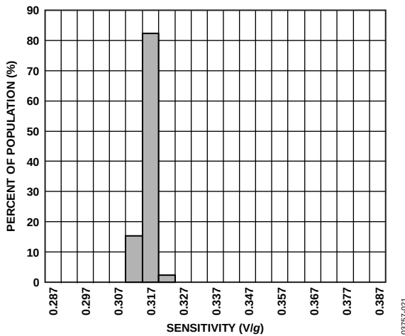
图21. 25°C时的X轴灵敏度
