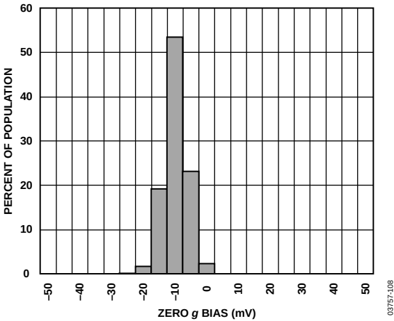
图28. 25°C时相对理想值的Y轴0 g偏置
