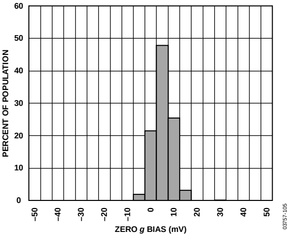
图25. 25°C时相对理想值的X轴0 g偏置
