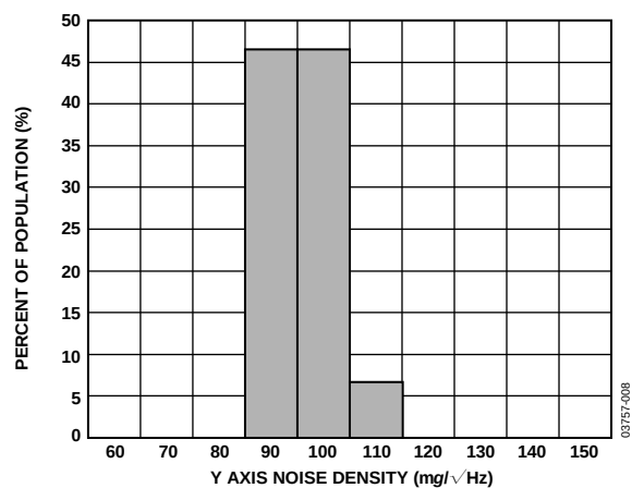
图14. 25°C时的Y轴噪声密度
