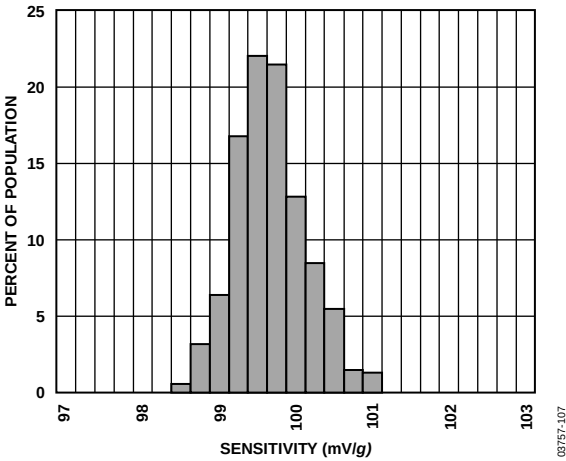
图27. 25°C时的X轴灵敏度
