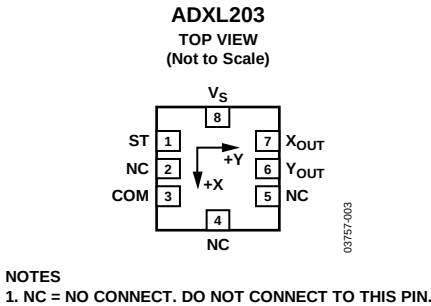
图4. ADXL203引脚配置
