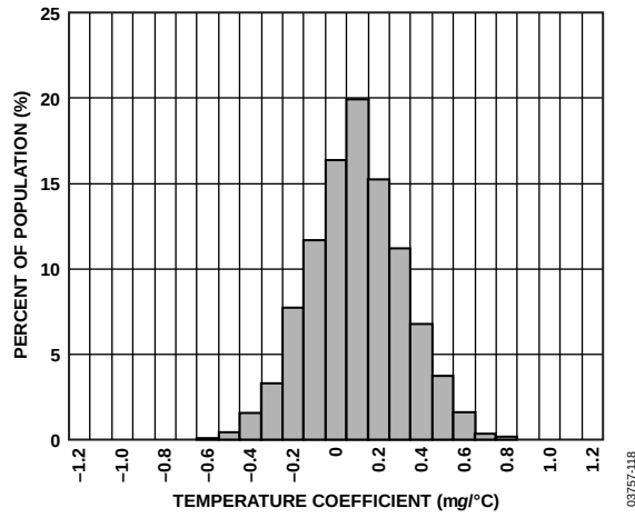
图20. X轴0 g偏置温度系数
