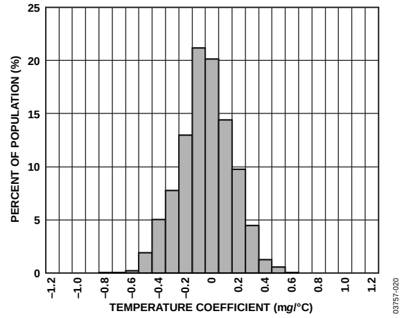
图23. Y轴0 g偏置温度系数
