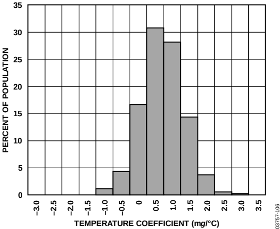
图26. X轴0 g偏置温度系数
