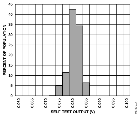
图33. 25°C时的Y轴自测响应
