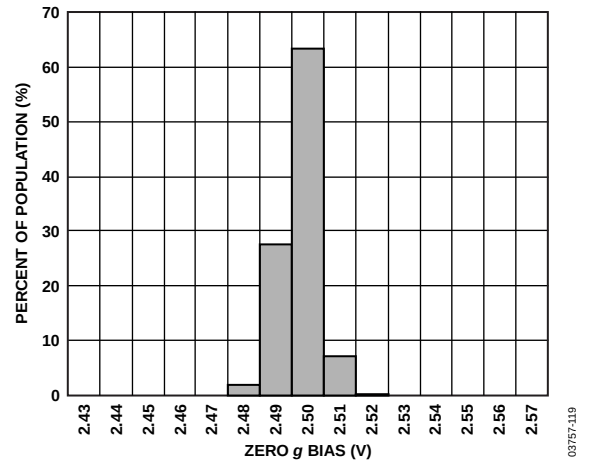
图22. 25°C时的Y轴0 g偏置
