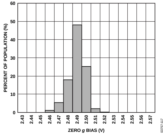
图19. 25°C时的X轴0 g偏置
