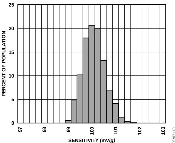
图30. 25°C时的Y轴灵敏度
