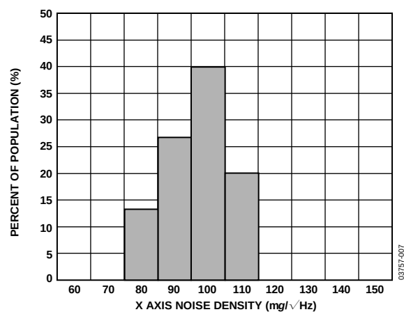
图12. 25°C时的X轴噪声密度
