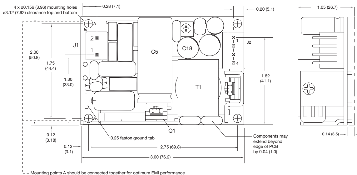
Output Connector J2 Molex PN 09-65-2048
